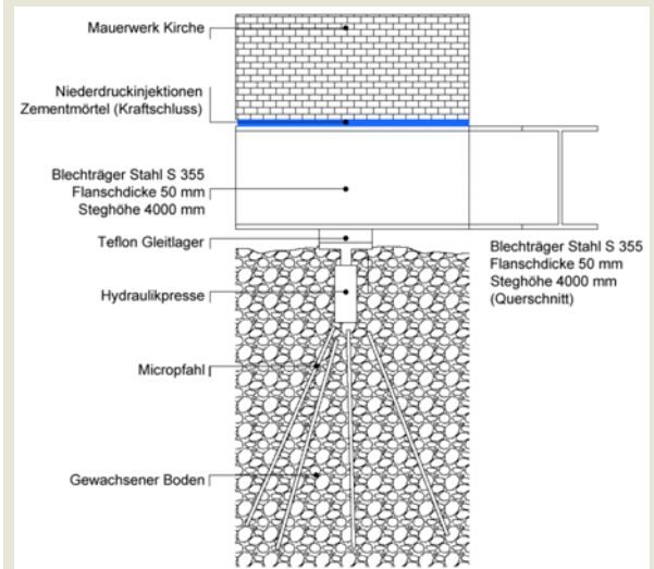
Abb. 3: Verschubkonzept mit Trägerrost, Pressen, Micropfählen (Ansicht)
